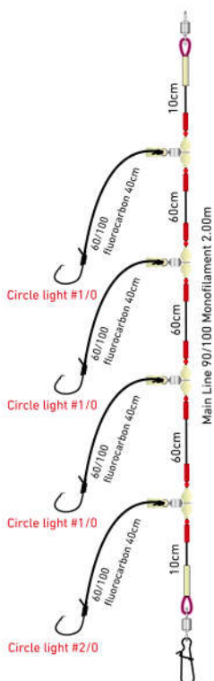
Montage Tanacom Pêche profonde Light
