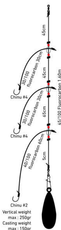
Montage Bateau compétition Light
