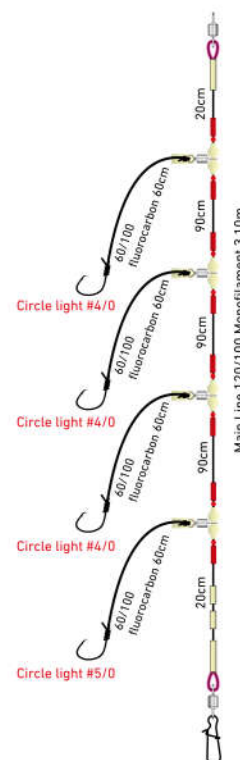
Montage Tanacom Pêche profonde Heavy
