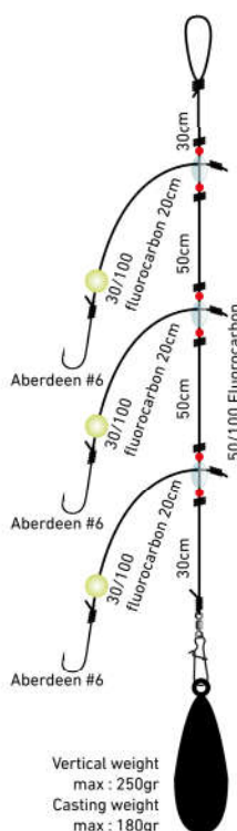
Montage Poissons plats
