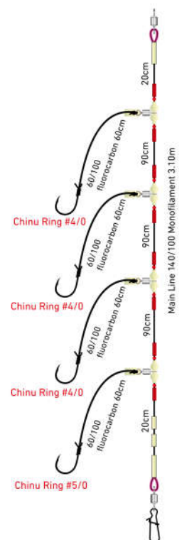
Montage Tanacom Pêche profonde Extra Heavy
