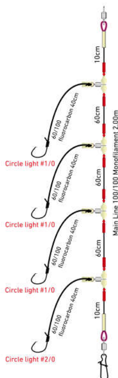
Montage Tanacom Pêche profonde Medium
