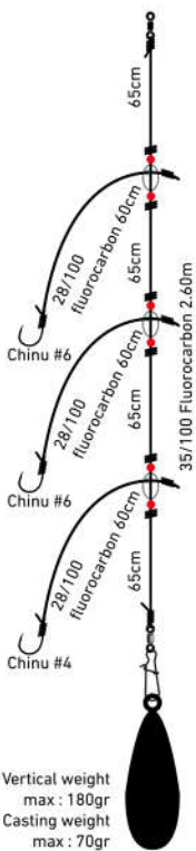
Montages Bateau compétition Shallow Depth Light
