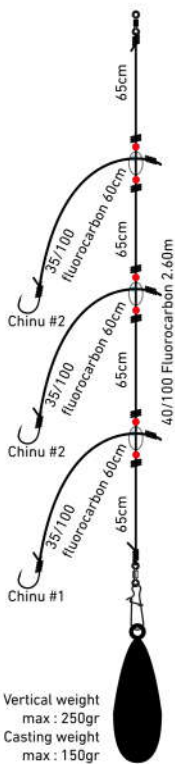
Montages Bateau compétition Shallow Depth Medium
