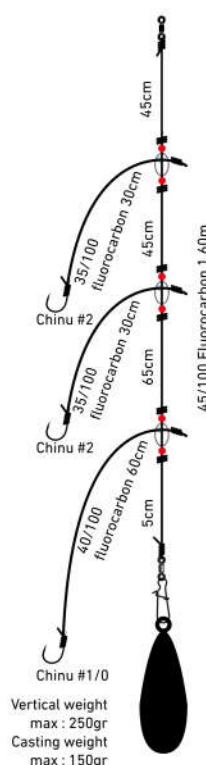
Montage Bateau compétition Heavy
