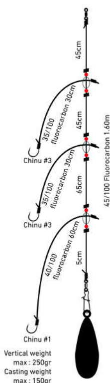
Montage Bateau compétition Medium
