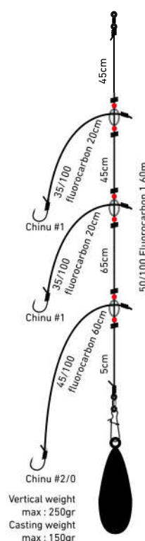
Montage Bateau compétition Extra Heavy
