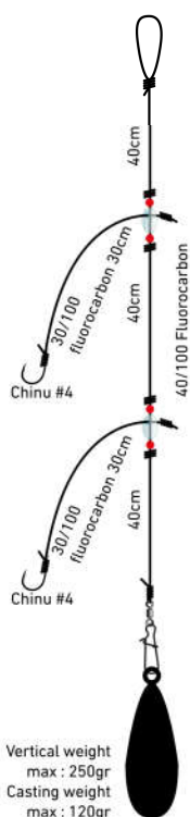
Montages Daurade Bateau
