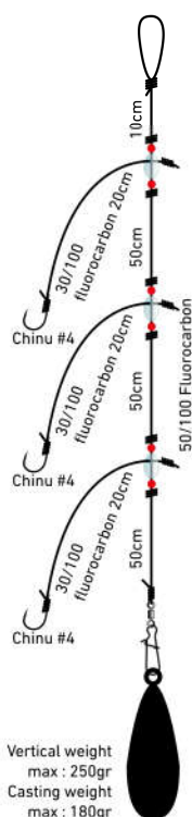
Montage Daurade Bord/Bateau
